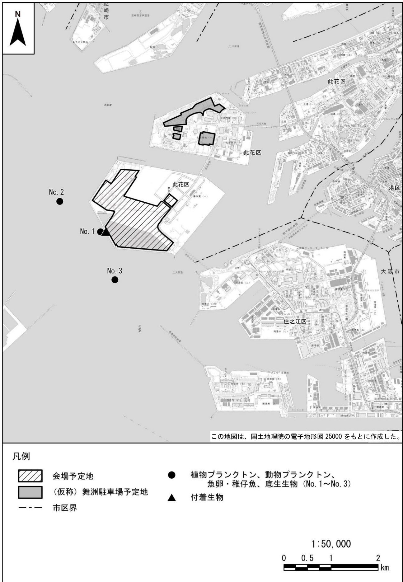
図 5.10.3(1) 現況調査地点 (海域動植物)
