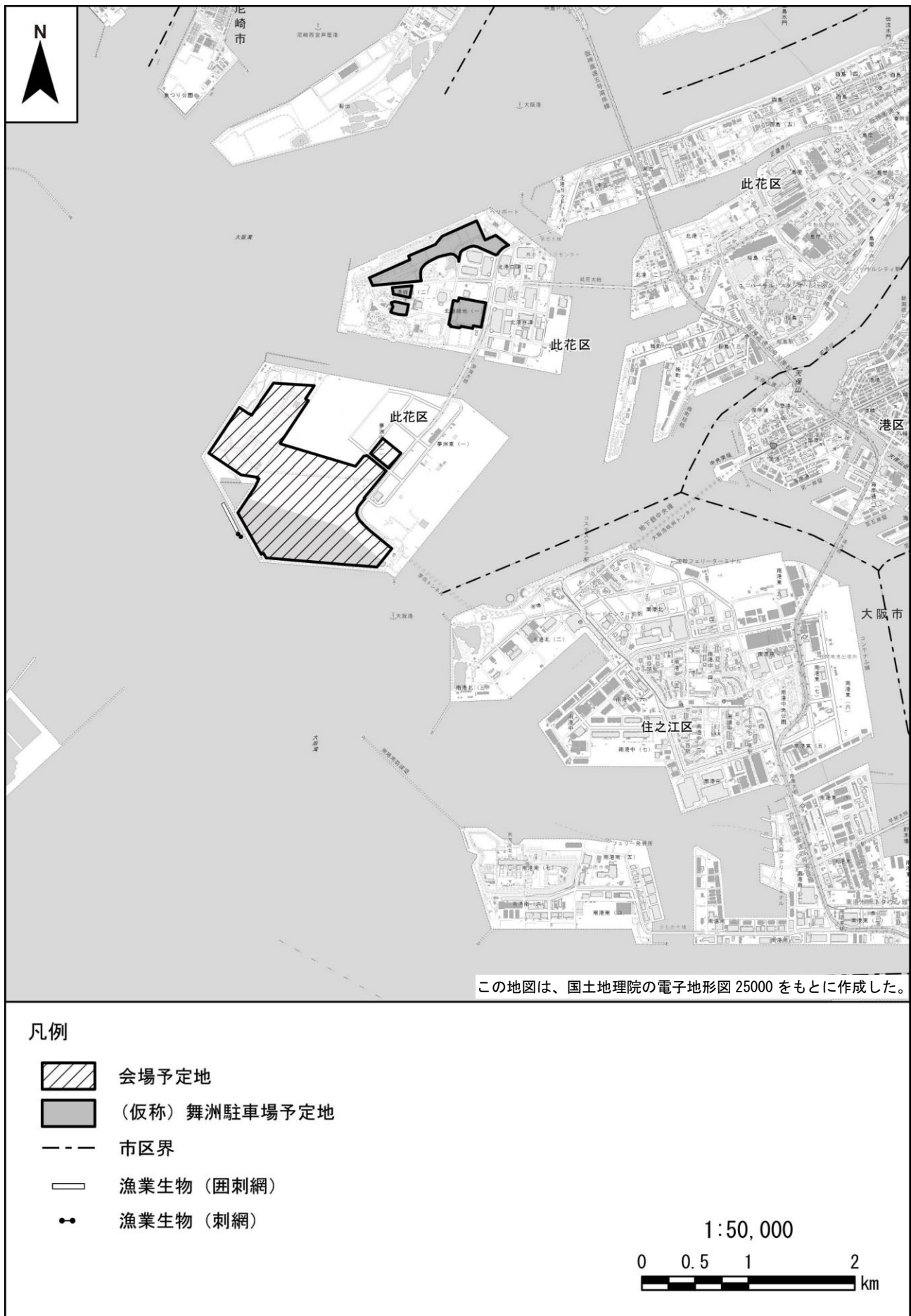
図 5.10.3(2) 現況調査地点 (海域動物)
