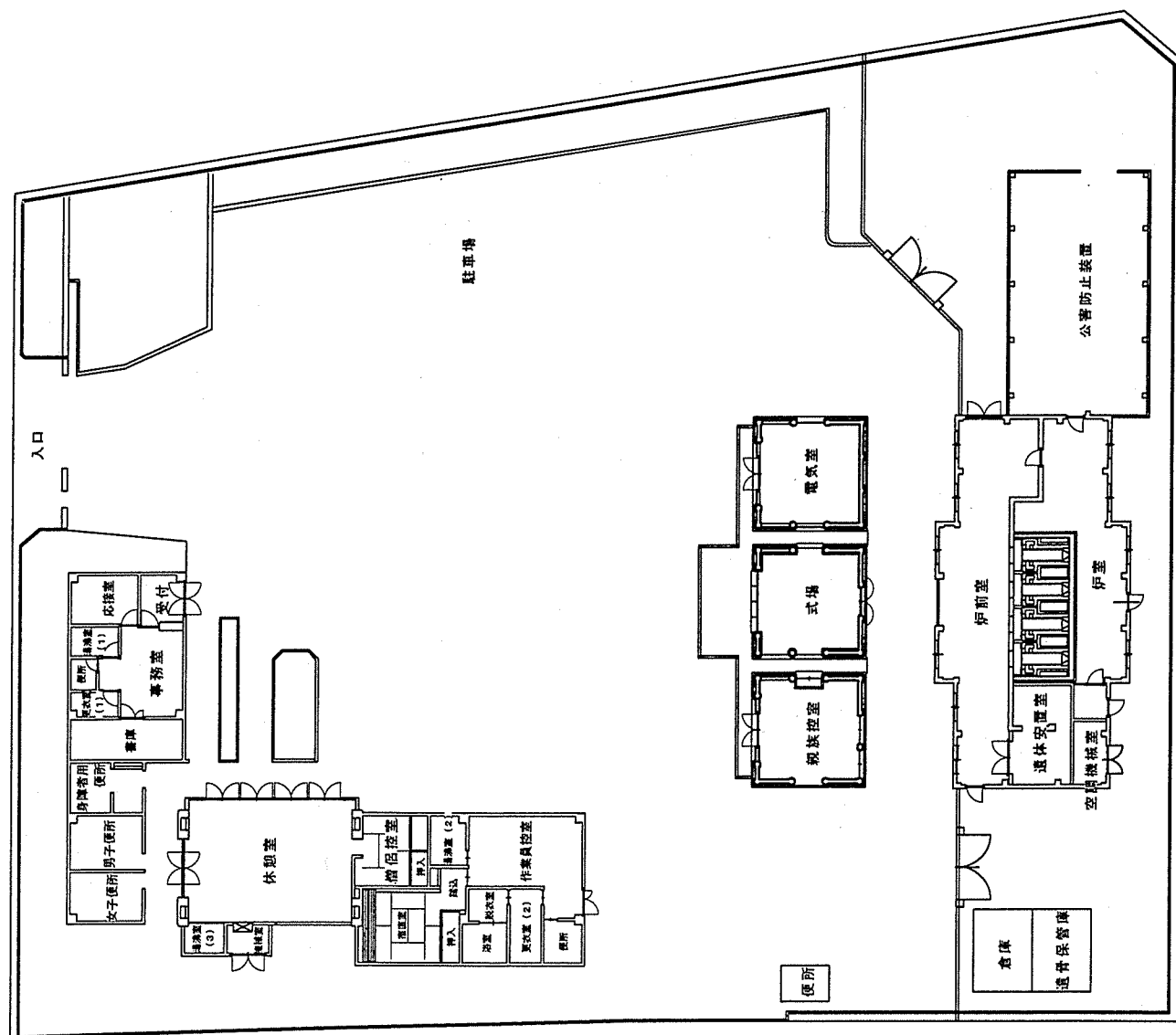
配置図・平面図
