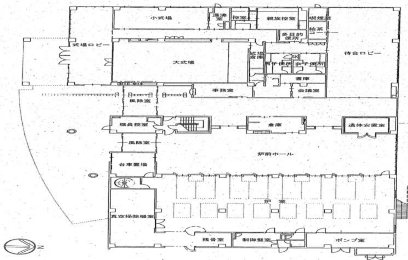
1 階平面図
