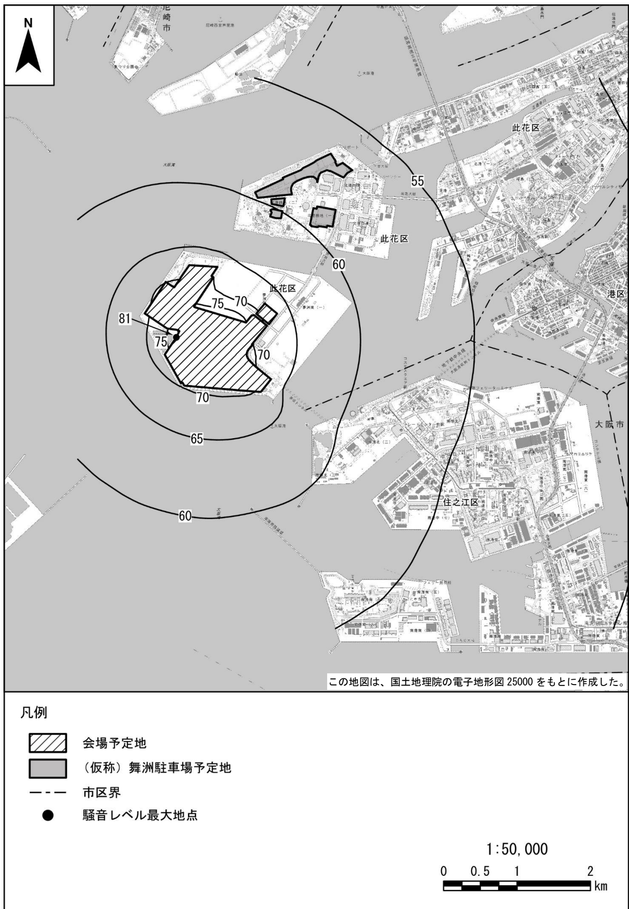
図 5.5.15(1) 建設機械騒音予測結果（会場予定地）
