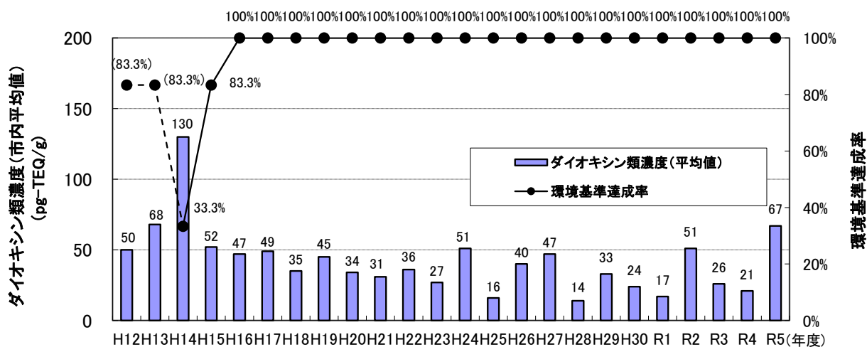
図7 ダイオキシン類常時監視結果の推移（海域底質）
