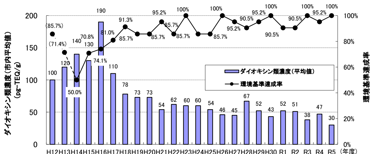
図6 ダイオキシン類常時監視結果の推移（河川底質）
