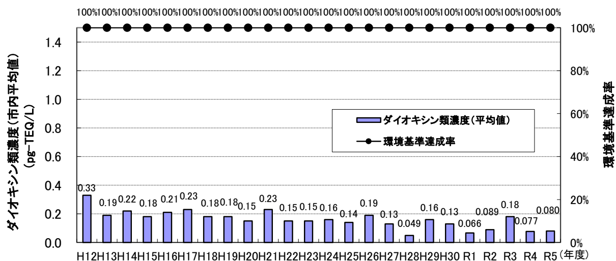
図4 ダイオキシン類常時監視結果の推移（海域水質）
