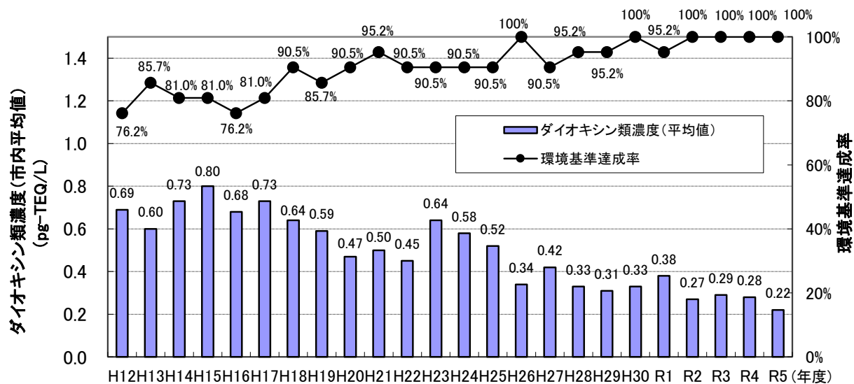
図3 ダイオキシン類常時監視結果の推移（河川水質）
