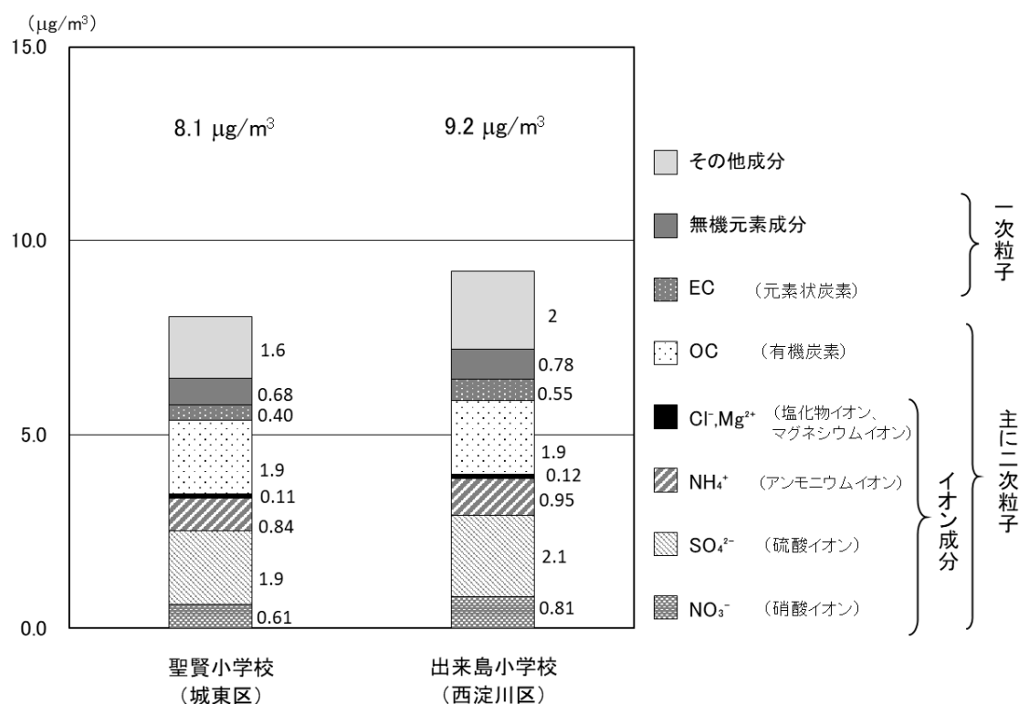
図3-3 微小粒子状物質の令和7年度における成分分析結果（年平均濃度）
