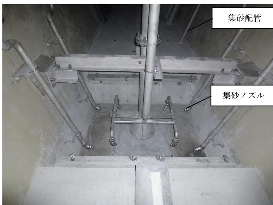
写真 3 揚砂ピット（閉塞防止用保護スクリーン下部）
