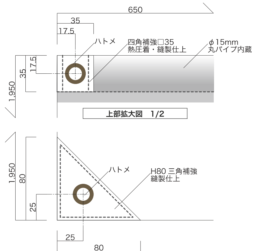
下部拡大図 1/2
