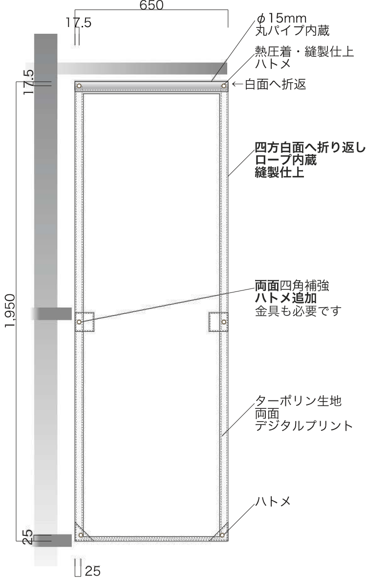
全体図 1/15
