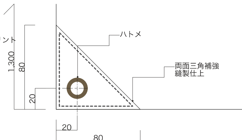
下部拡大図 1/2
