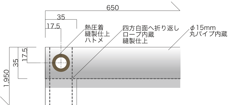
上部拡大図 1/2
