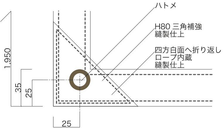
下部拡大図 1/2
