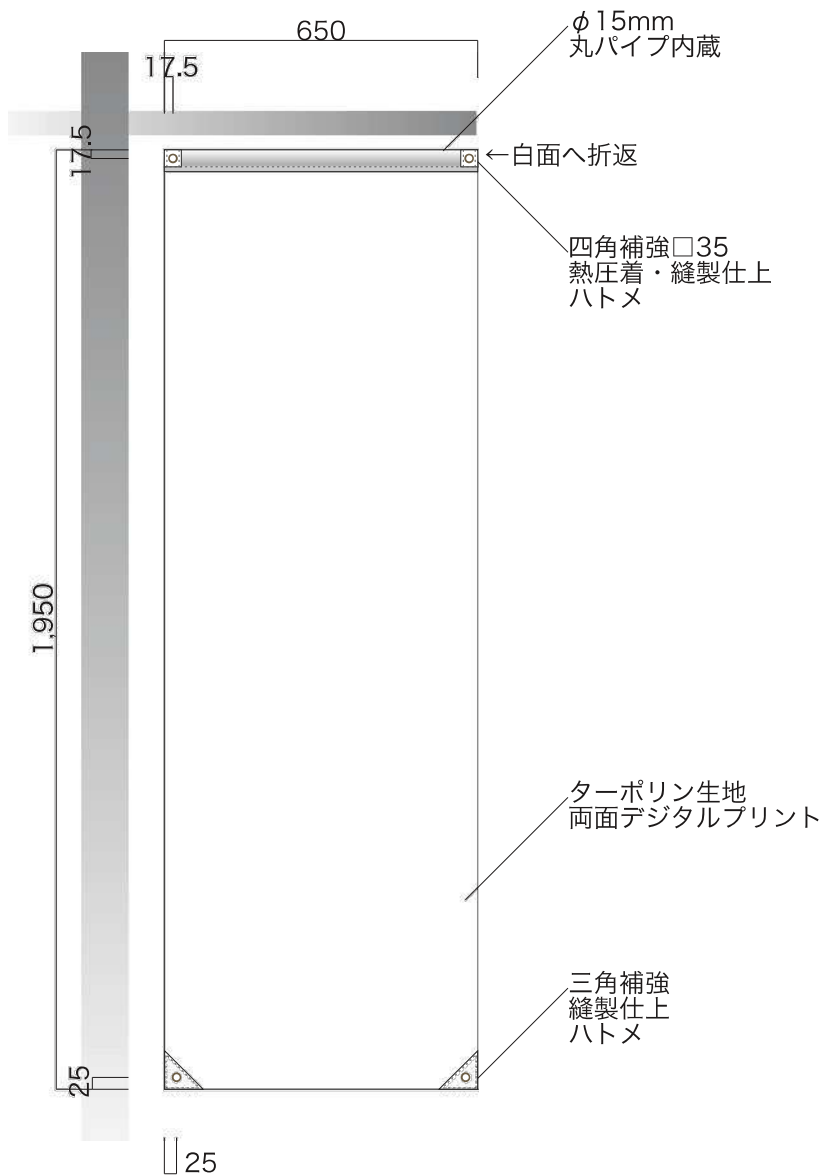
全体図 1/15
