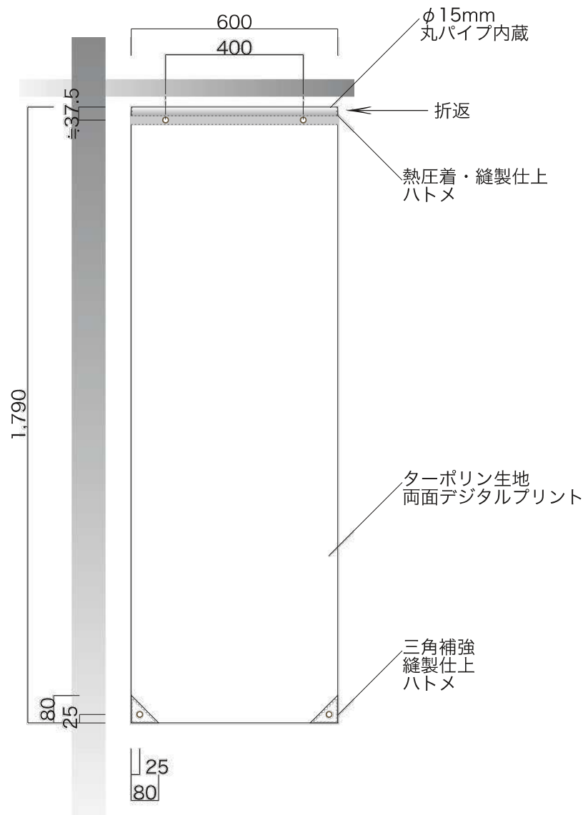
全体図 1/15
