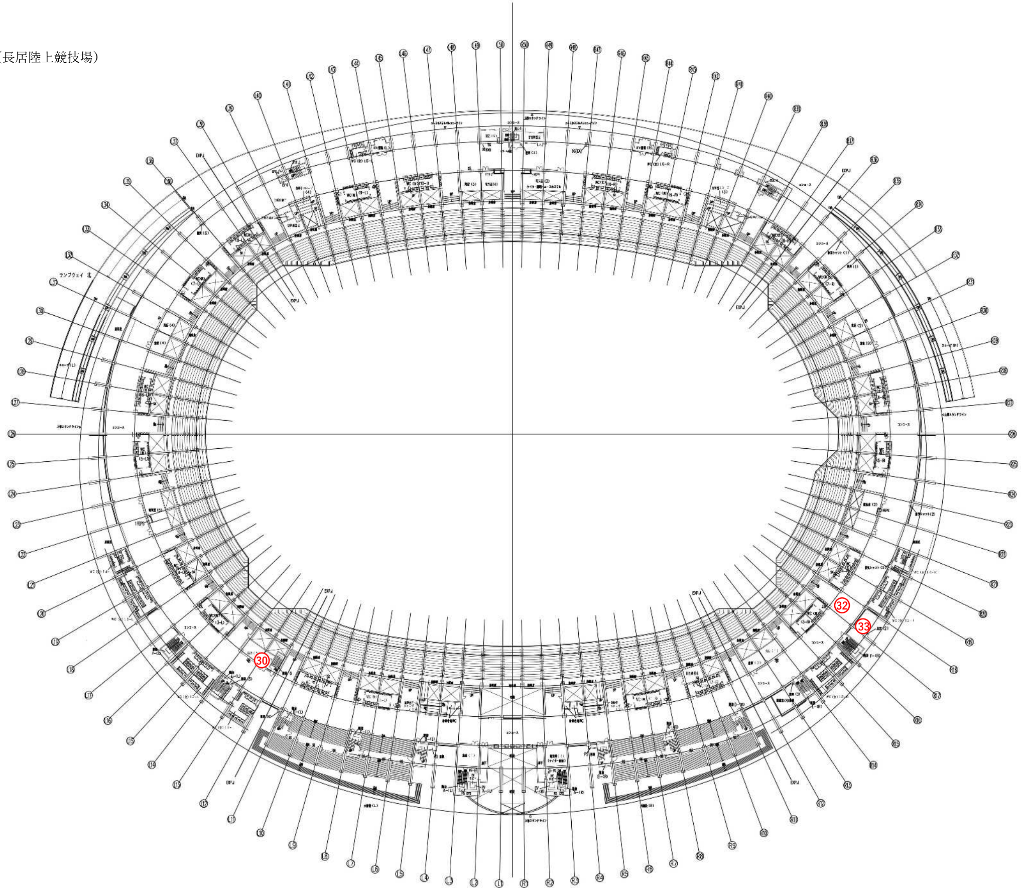
2階平面図
