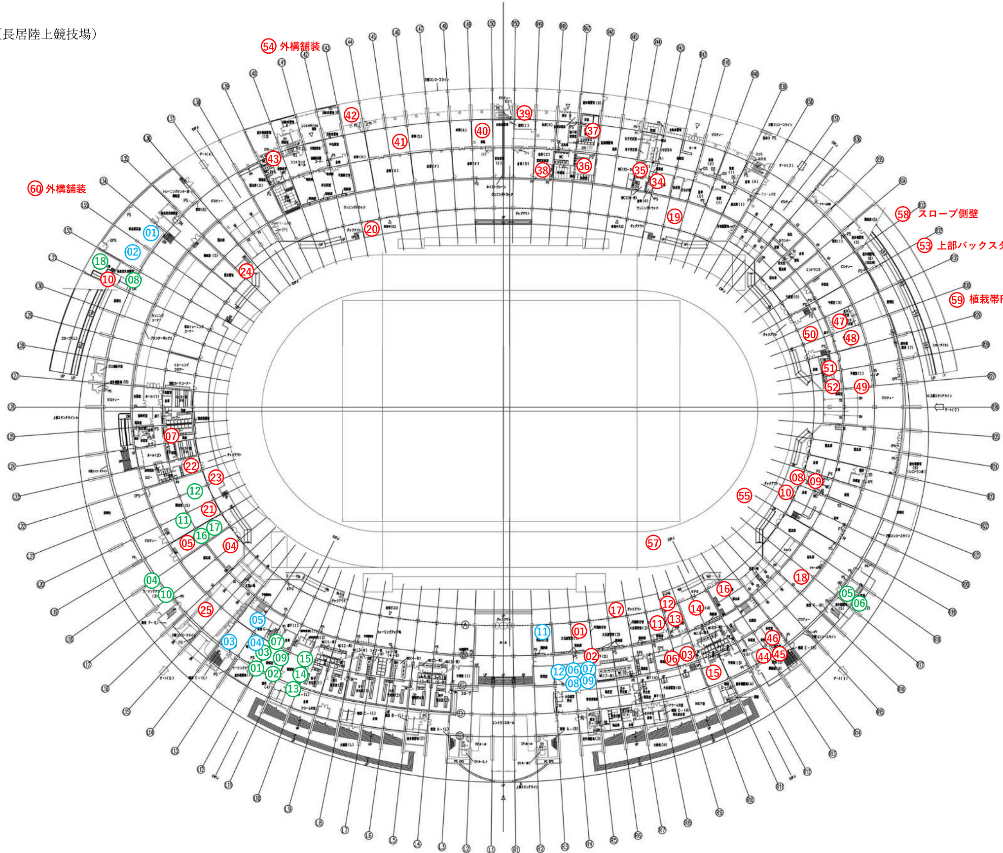
1 階平面図
