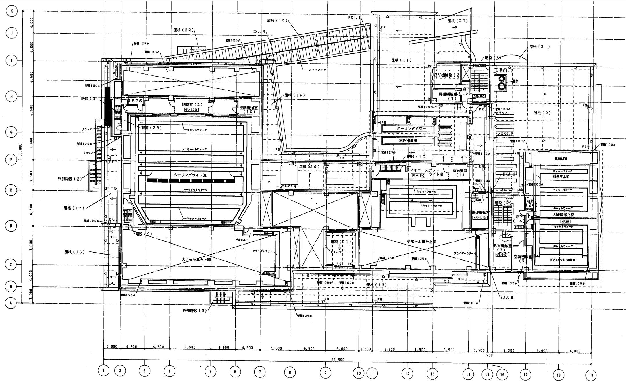
4階平面図
