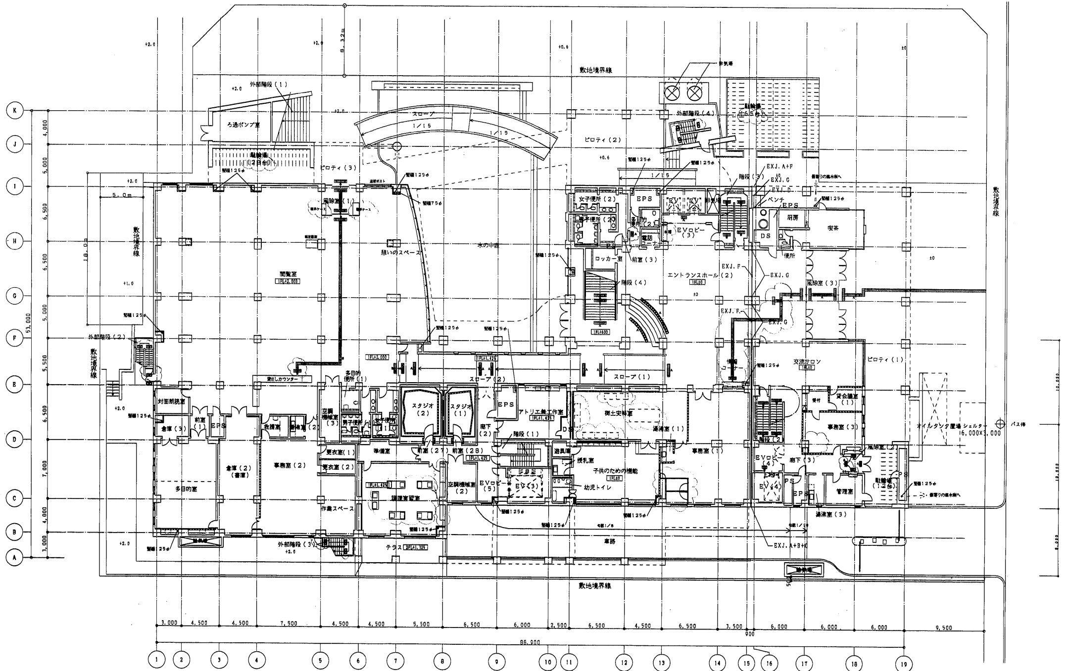
1階平面図
