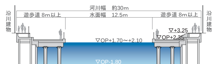
●遊歩道一般区間断面図
