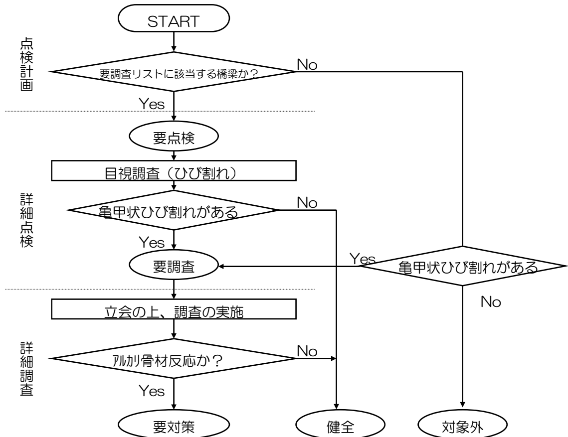
図-1.8 アルカリ骨材反応調査のフロー
