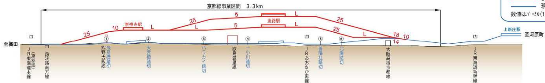
京都線縦断面図
