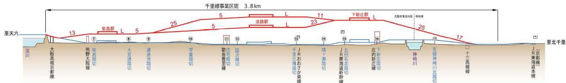
千里線縦断面図
