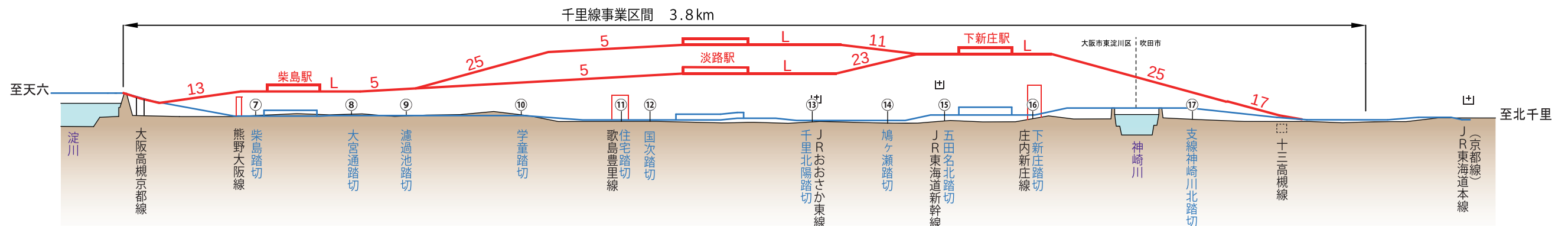
千里線縦断面図
