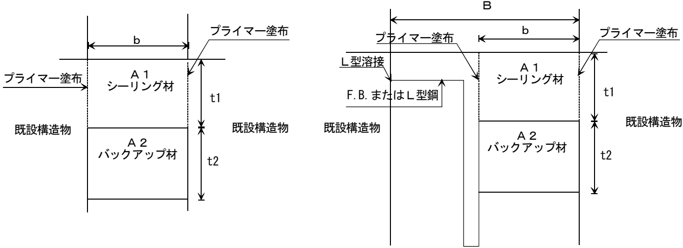
2-1 標準施工断面
