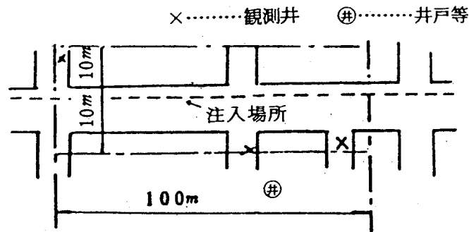
図-4 観測井の設置平面図 (参考)
