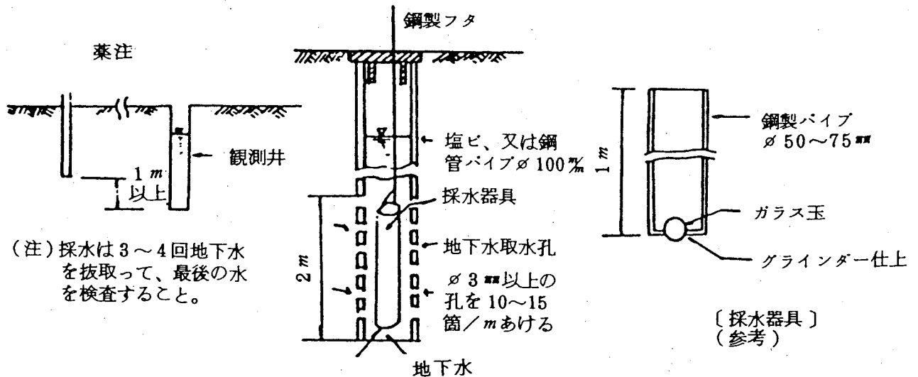
図-5 観測井の構造図 (参考)
