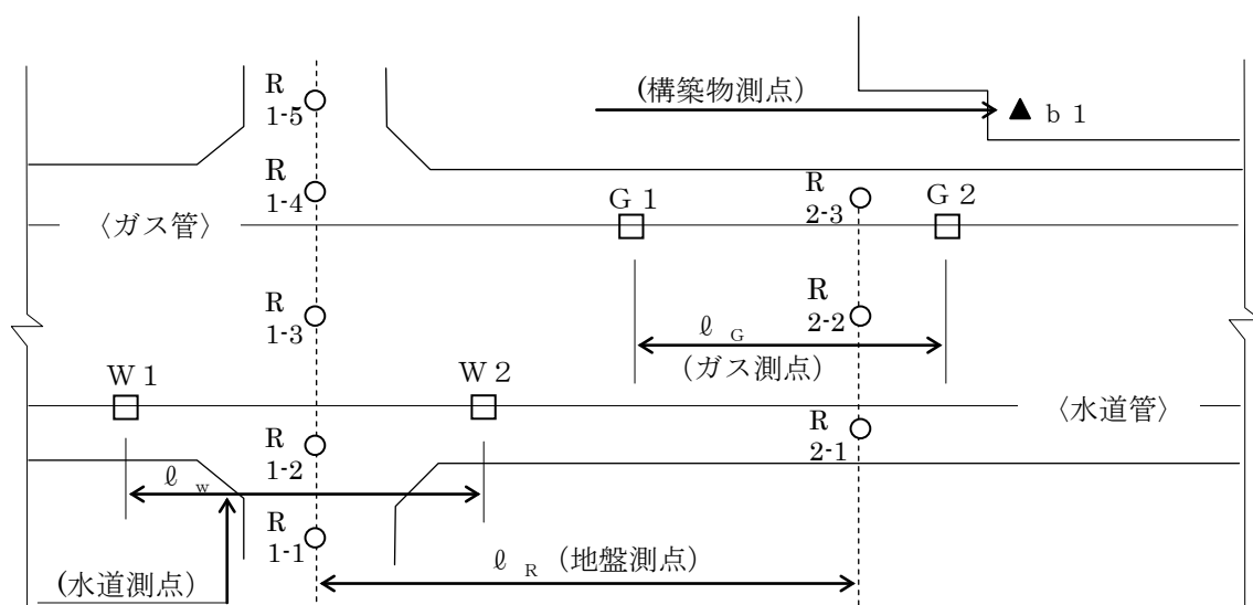
図－４ 観測孔及び観測点平面図（作成例）
