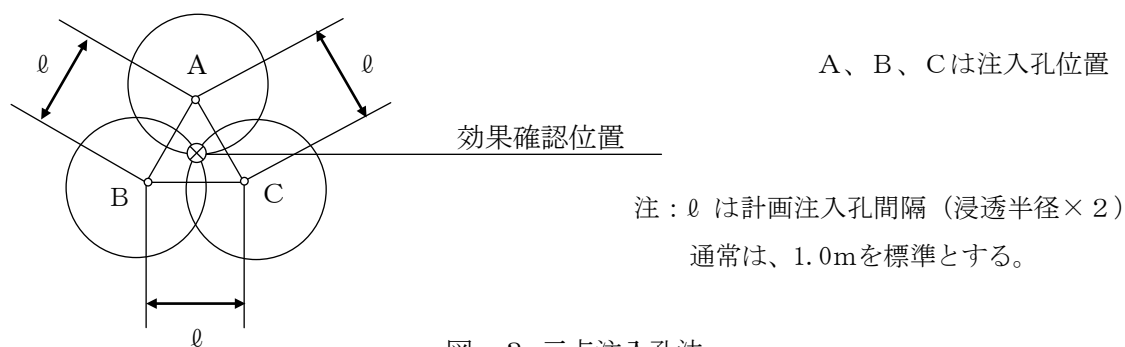
図－３ 三点注入孔法
