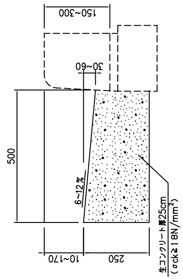
街渠 コンクリート L・A交通 (路盤なし)
