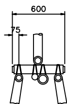
3本鳥居型支柱平面図
