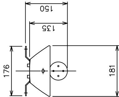
A 矢 視 図
