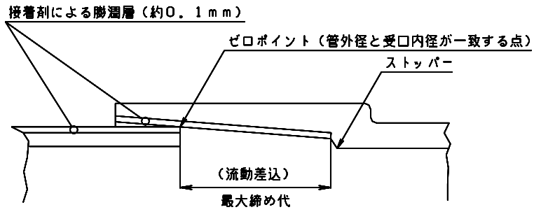
図-1 TS接合の原理
