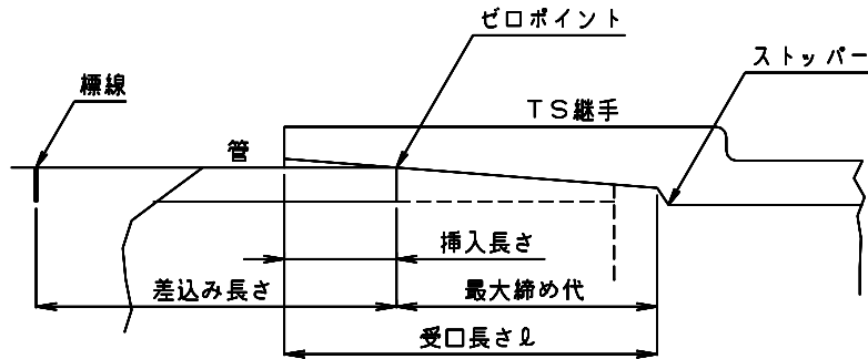
図-2 ゼロポイントと締め代
