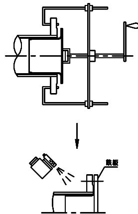
図-1 ねじ込・溶接フランジ
