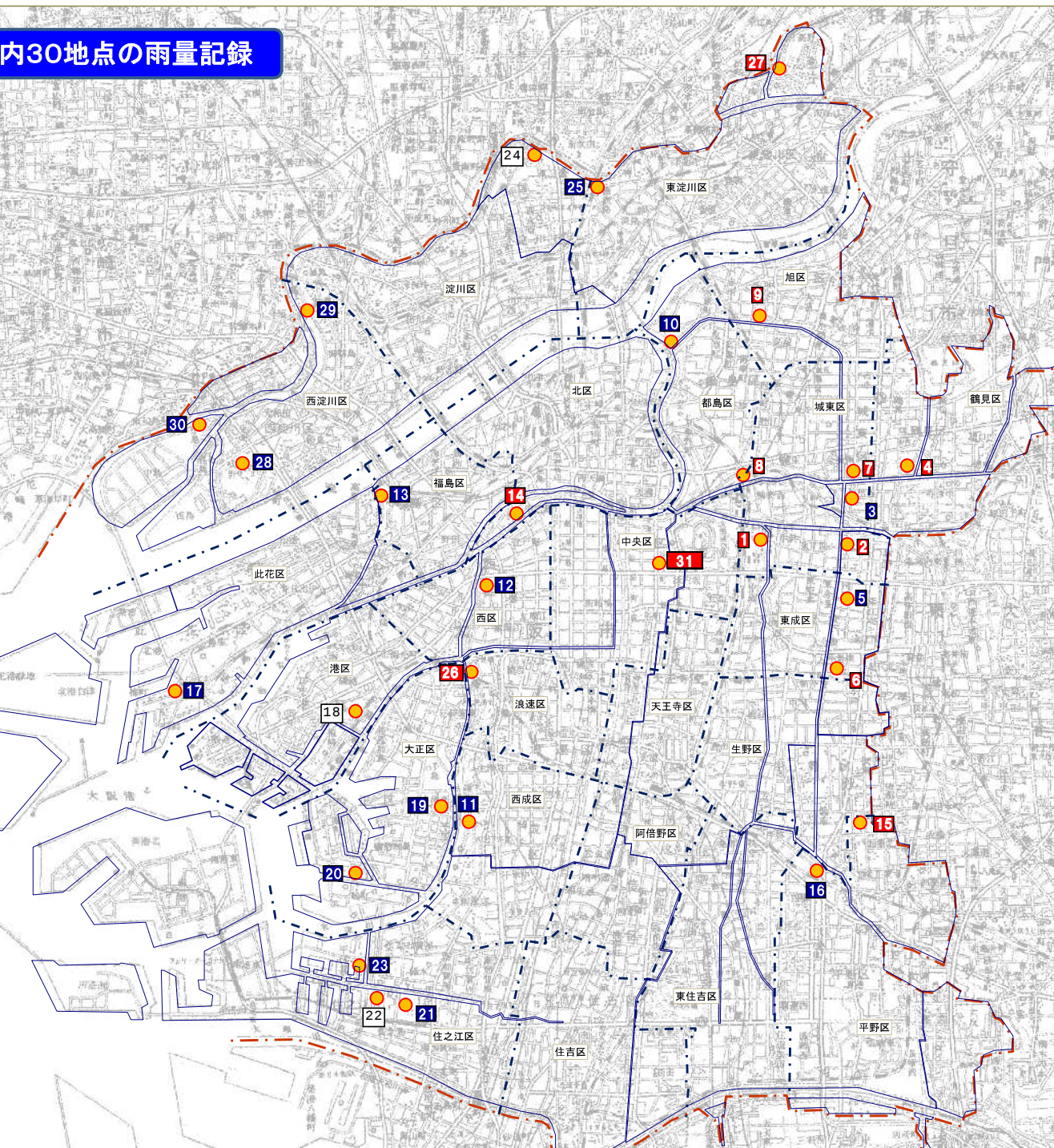
平成23年8月27日豪雨の大阪市内雨量記録
