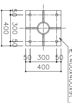
③-③ 断面
