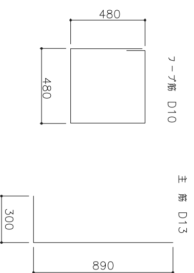
鉄筋加工図
