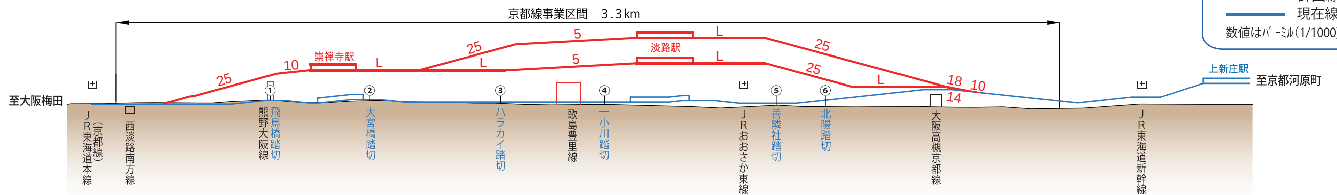
京都線縦断面図
