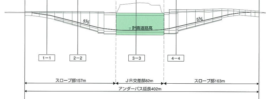
縦断面図
