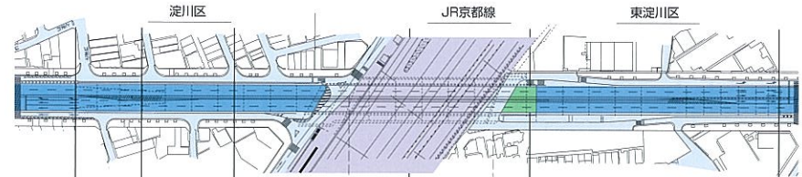
平面図
