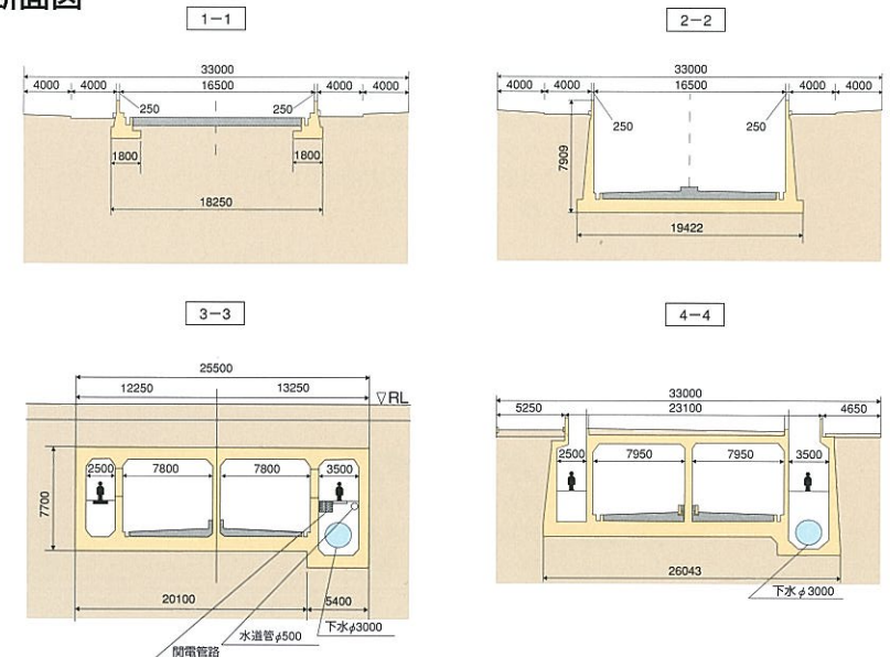
横断面図
