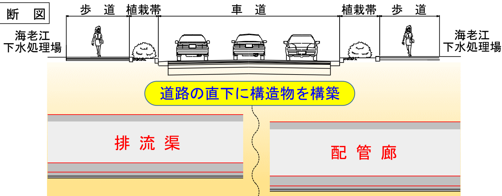
横断図
