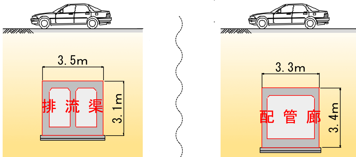
横断図
