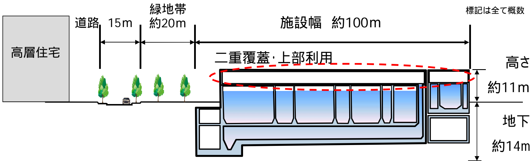
水処理施設配置イメージ
