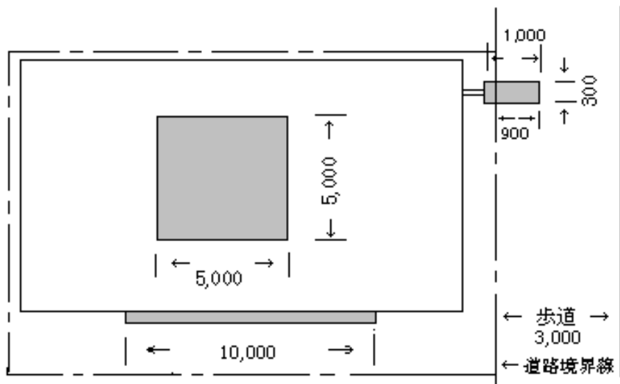
【平面図の例】
