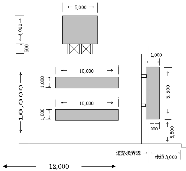
【立面図の例】
