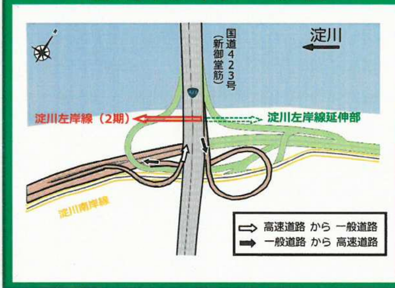
豊崎ICイメージ図
