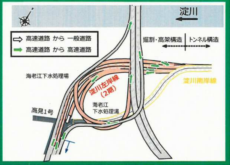
海老江JCTイメージ図
