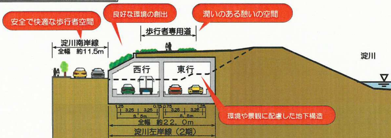
淀川左岸線 (2期) 断面イメージ
