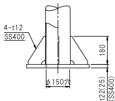
柱脚部詳細
