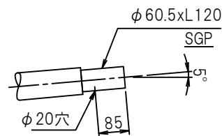
アダプタ-詳細
