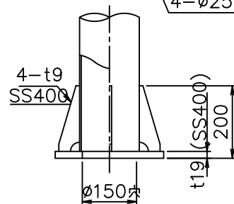
柱脚部詳細
