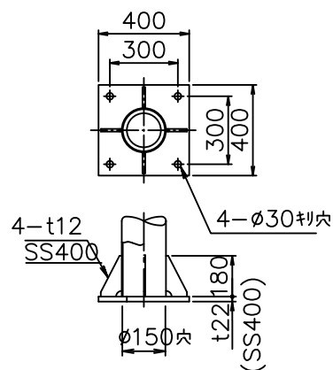
柱脚部詳細 8M用
