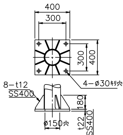
柱脚部詳細 10M用
