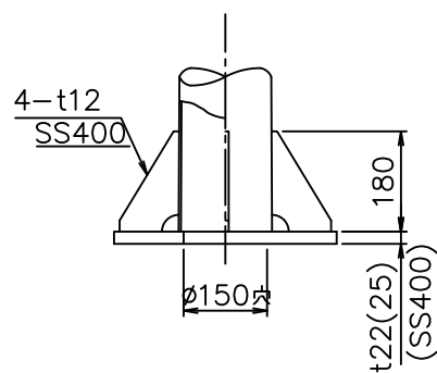
柱脚部詳細
