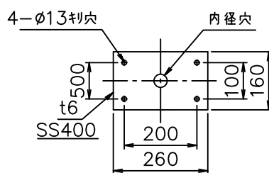
器具取付フランジ詳細
