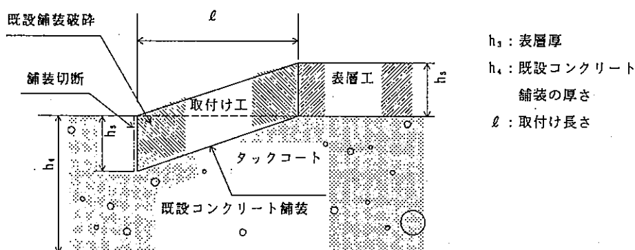
図 3-9-1 既設舗装取付け詳細図
