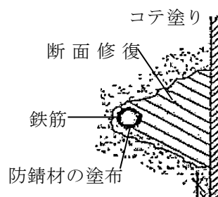
図 3－9－2 断面修復工
