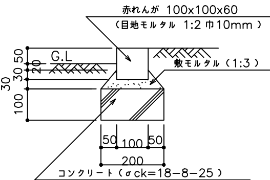
レンガ縁石（A）
