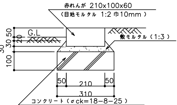
レンガ縁石（C）
