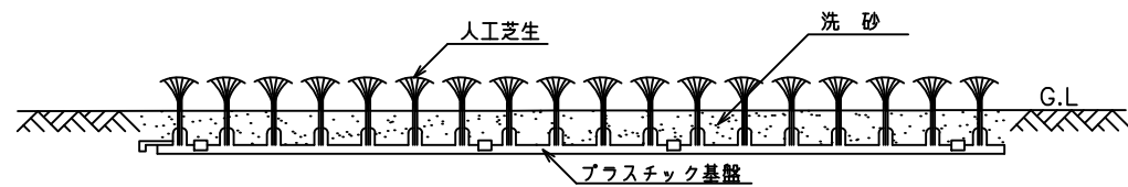
右側面図
