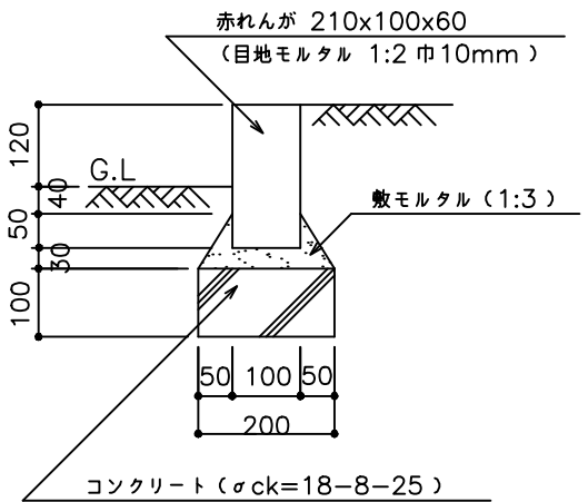
レンガ縁石（B）
