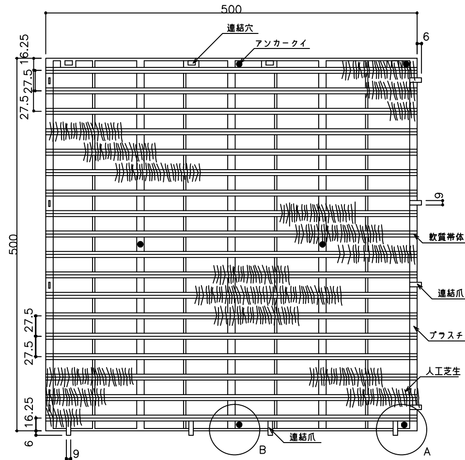
立面図
