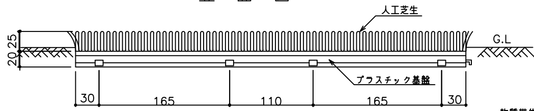
立面図
