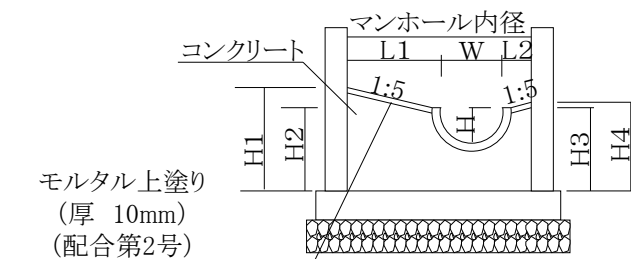
断面図
