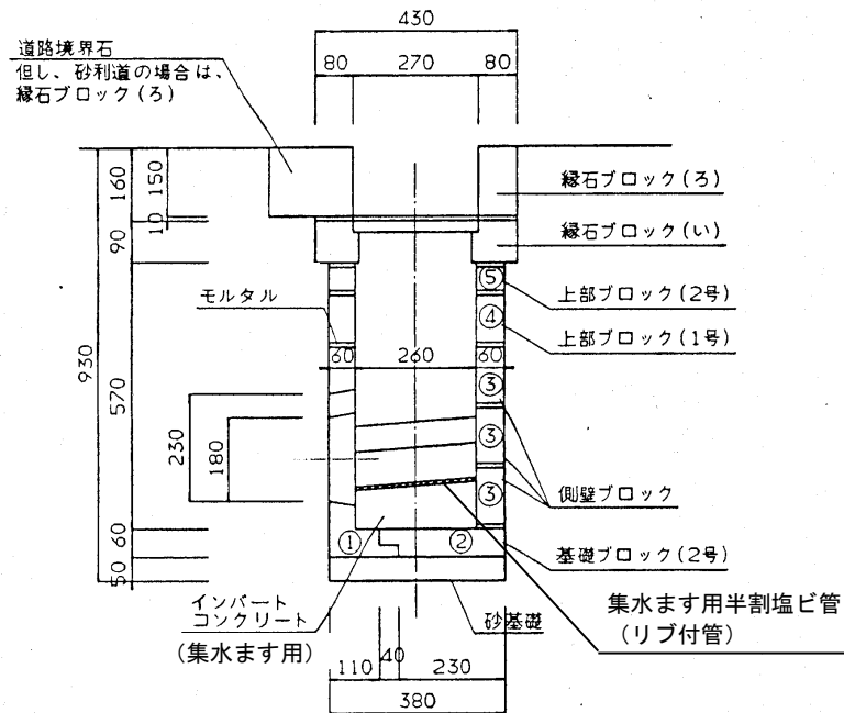
側面（断面）図
