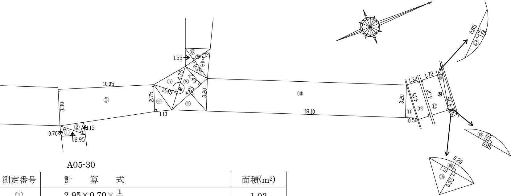
二次復旧工 舗装面積図（例）
