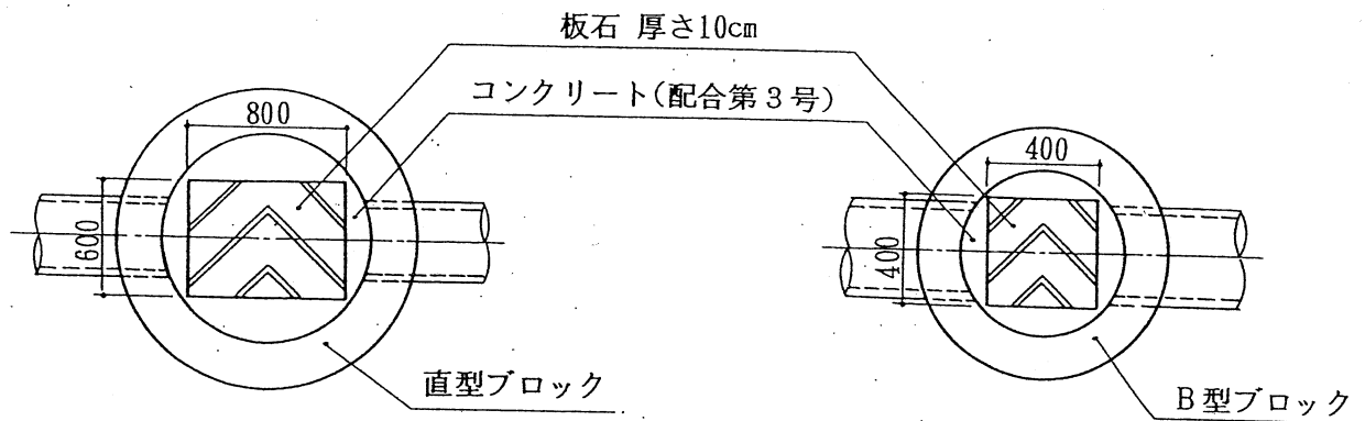
断面図
