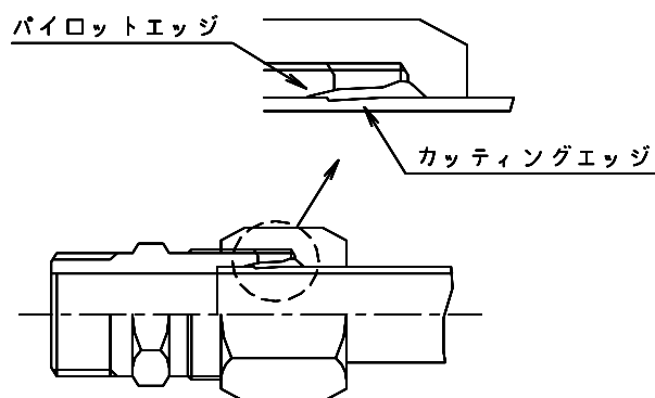
くい込継手
