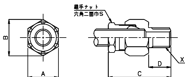
スリーブ継手
