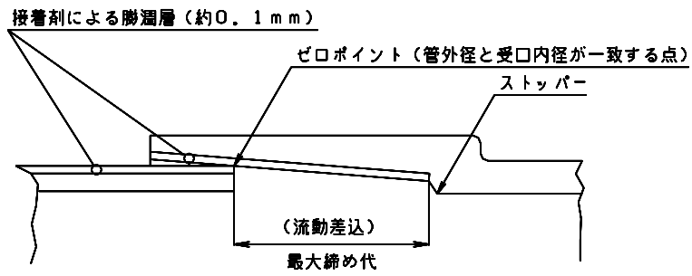
図ー1 TS接合の原理
