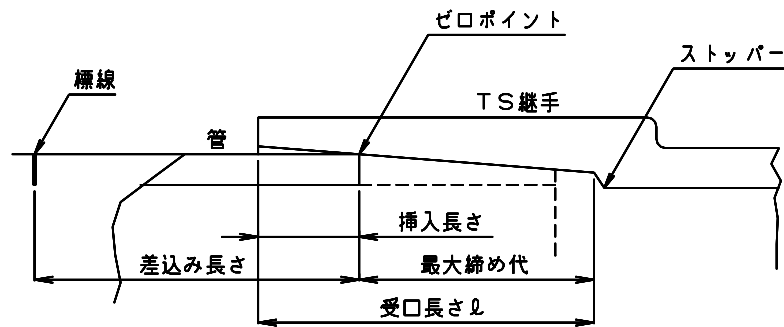
図ー2 ゼロポイントと締め代
