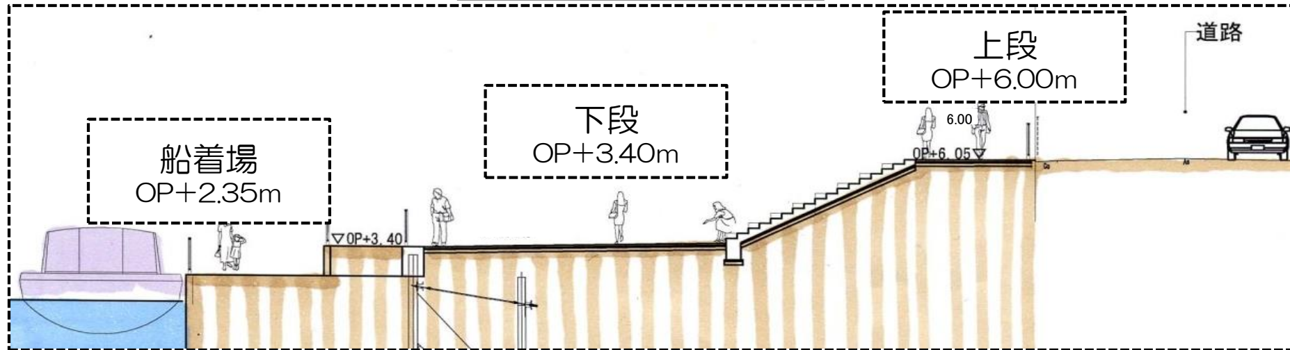
本町橋船着場付近断面図
