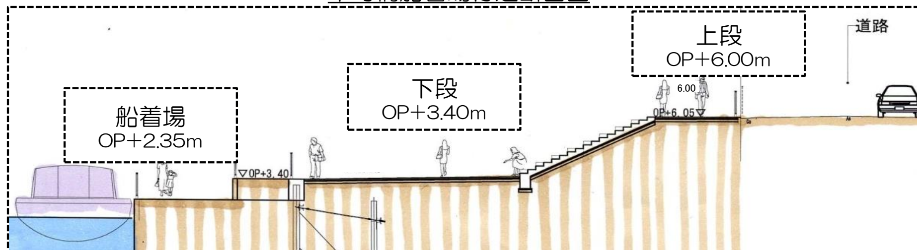
本町橋船着場付近断面図
