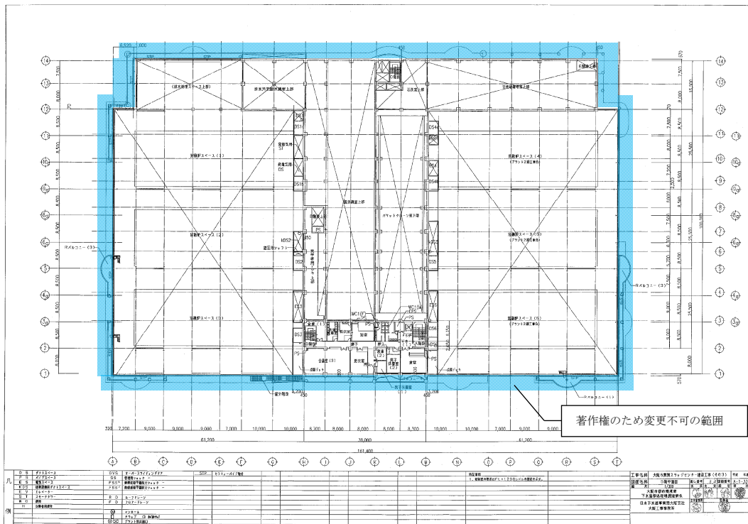
図 7-1 2 取合位置図 (舞洲スラッジセンター5F 平面図)
