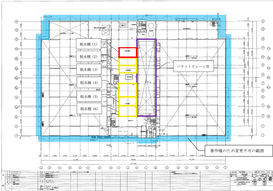
図 7-1 1 取合位置図 (舞洲スラッジセンター4F 平面図)
