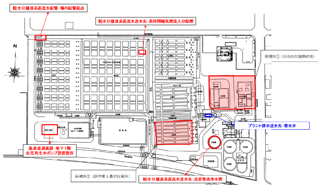
図 7-1 5 取合位置図 (此花下水処理場)
