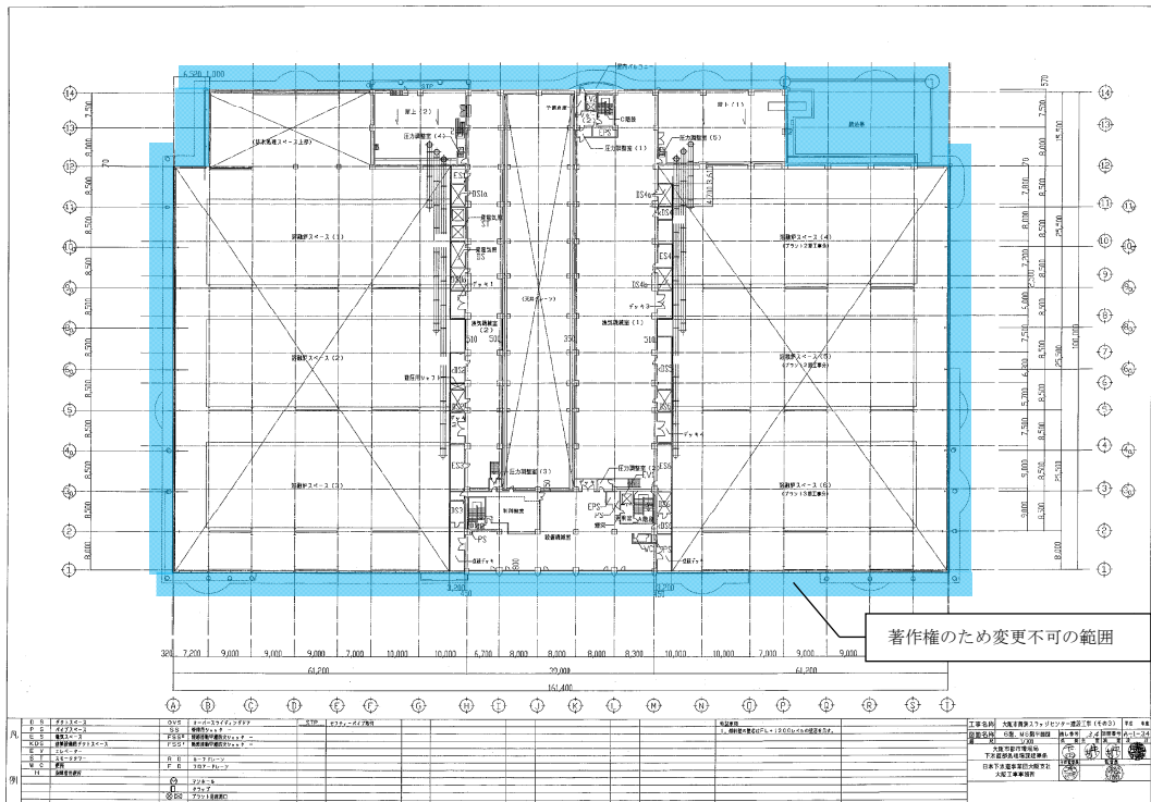
図 7-13 取合位置図 (舞洲スラッジセンター6F 平面図)
