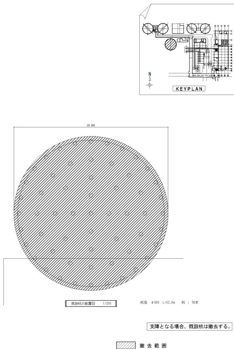
図 7-18 既設消化タンク杭の配置図
