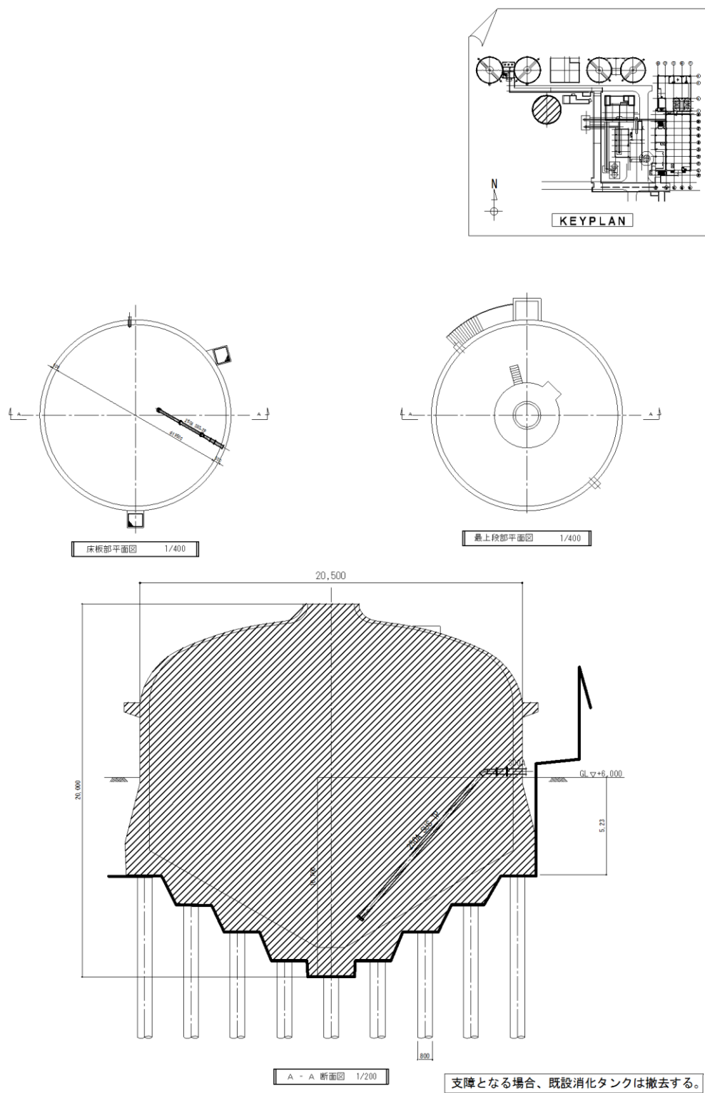
図 7-17 既設消化タンク本体の撤去図
