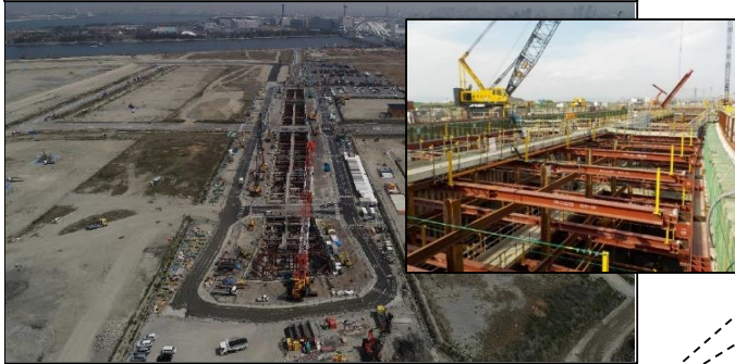
【10】鉄道駅舎建設工事の状況
