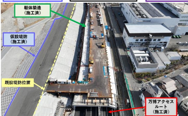
▲ 1 工区（国道 2 号～JR 神戸線）の工事状況（R7.2 月）
