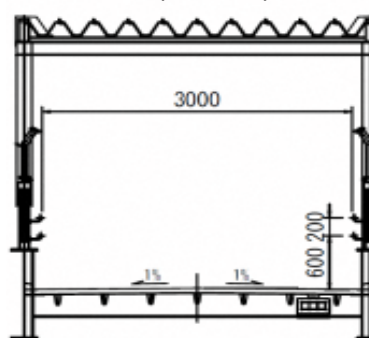
歩道橋(一般部)断面図
