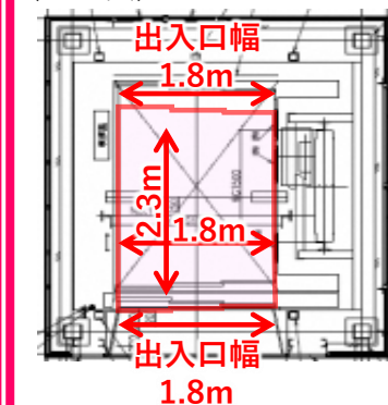
片側ドア同型設置事例(川西市)
