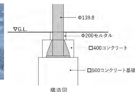
構造図
