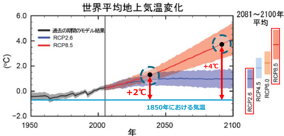
図2-5 1986-2005年平均に対する世界平均地上気温の変化
