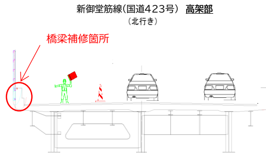
夜間工事 新御堂筋線(国道423号) 高架部 車線規制イメージ図
