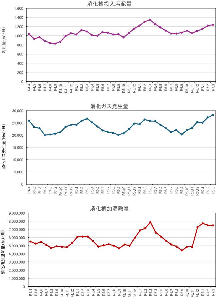
図 4-1 汚泥消化に係る実績値
