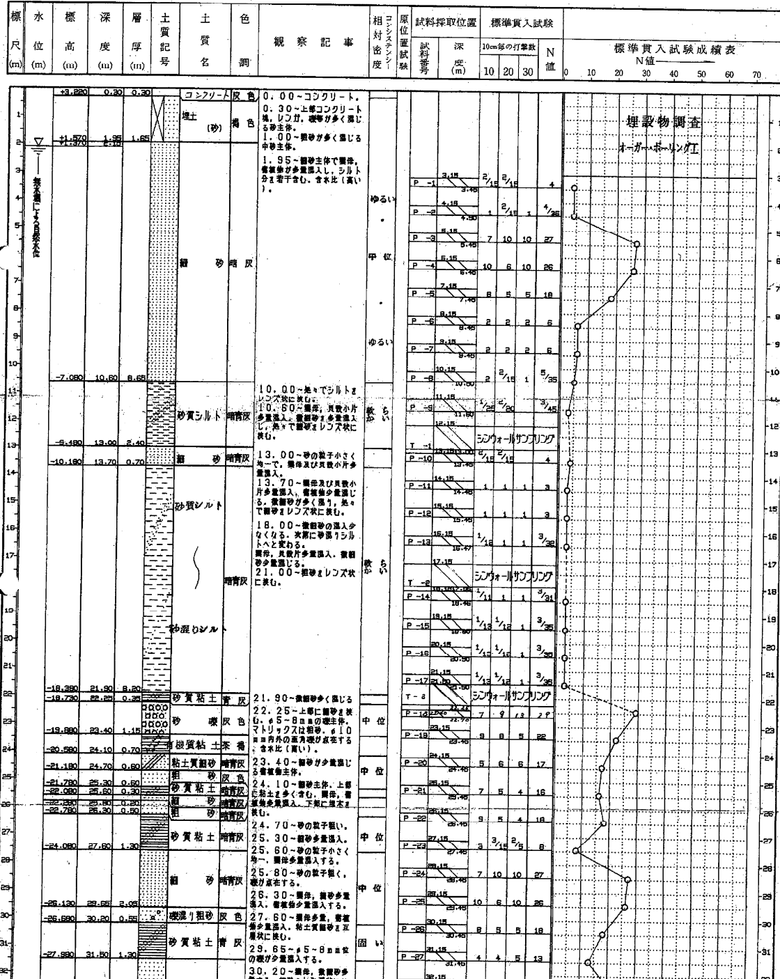
図 4-3 柱状図 No.1 (1/2)
