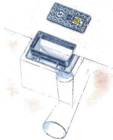
汚水受入れ ます 設置姿図
